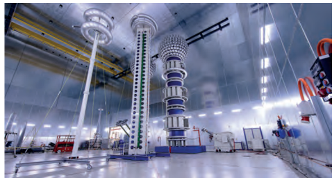
Bild 4: Stossspannungsgenerator zur Prüfung des Stosspannungsverhaltens der Kabel.
