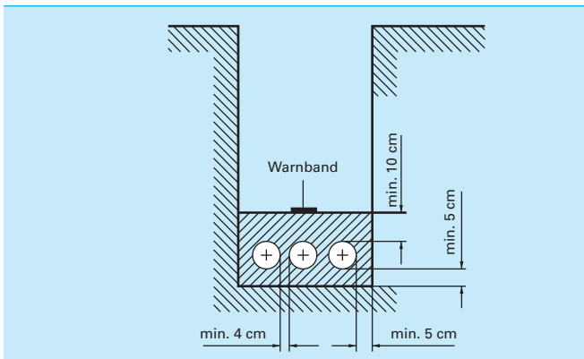
einlagig
